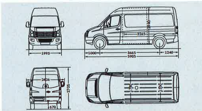
Crafter 30/35 Kastenwagen mittlerer Radstand mit Hochdach
