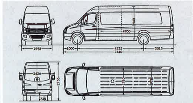
Crafter 50 Kastenwagen langer Radstand mit Überhang mit Hochdach
