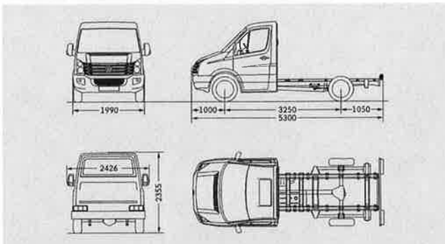
Crafter 35 Fahrgestell mit Einzelkabine kurzer Radstand
