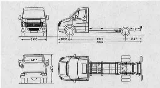
Crafter 50 Fahrgestell mit Einzelkabine langer Radstand
