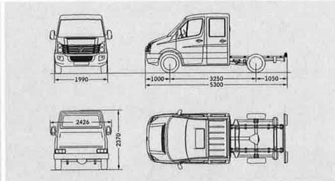
Crafter 35 Fahrgestell mit Doppelkabine kurzer Radstand
