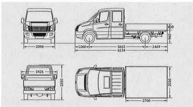
Crafter 35 Pritschenwagen mit Doppelkabine mittlerer Radstand
