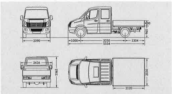
Crafter 30 Pritschenwagen mit Doppelkabine kurzer Radstand
