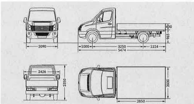
Crafter 30 Pritschenwagen mit Einzelkabine kurzer Radstand
