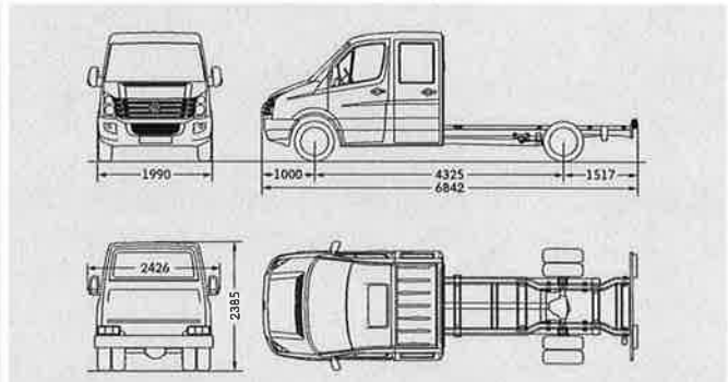
Crafter 50 Fahrgestell mit Doppelkabine langer Radstand
