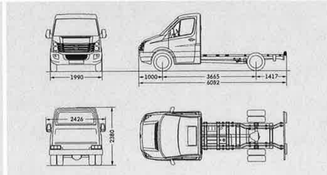
Crafter 50 Fahrgestell mit Einzelkabine mittlerer Radstand
