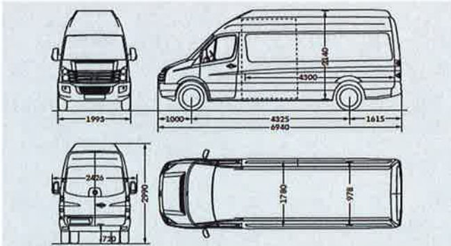
Crafter 50 Kastenwagen langer Radstand mit Superhochdach
