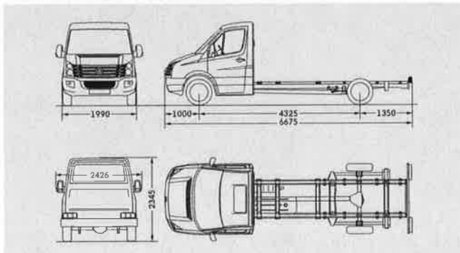
Crafter 35 Fahrgestell mit Einzelkabine langer Radstand
