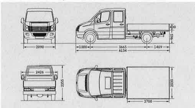
Crafter 30 Pritschenwagen mit Doppelkabine mittlerer Radstand
