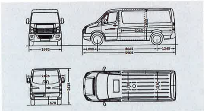
Crafter 30/35 Kastenwagen mittlerer Radstand mit Normaldach
