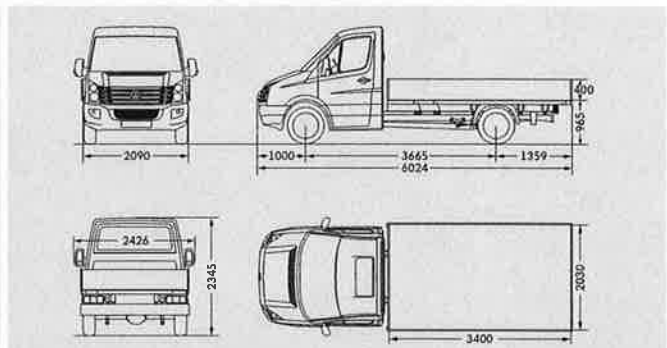
Crafter 30 Pritschenwagen mit Einzelkabine mittlerer Radstand
