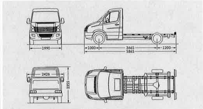
Crafter 30 Fahrgestell mit Einzelkabine mittlerer Radstand
