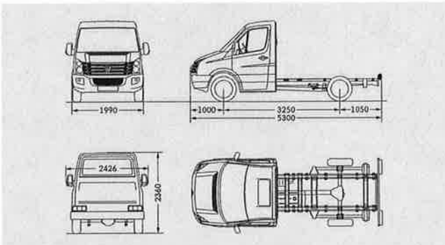
Crafter 30 Fahrgestell mit Einzelkabine kurzer Radstand
