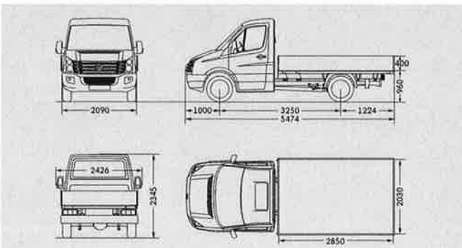
Crafter 35 Pritschenwagen mit Einzelkabine kurzer Radstand
