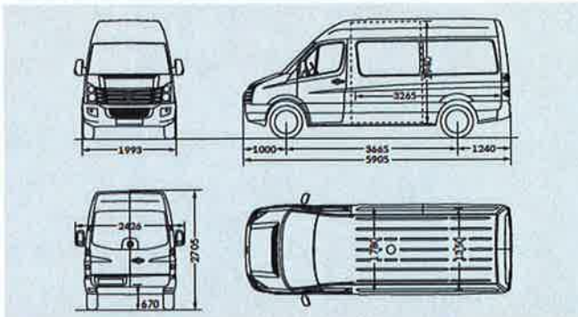
Crafter 30/35 Kombi mittlerer Radstand mit Hochdach
