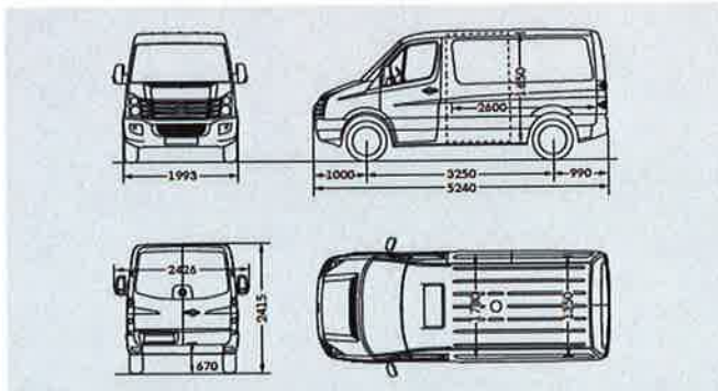
Crafter 30/35 Kastenwagen kurzer Radstand mit Normaldach
