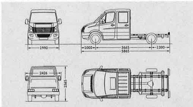
Crafter 30 Fahrgestell mit Doppelkabine mittlerer Radstand
