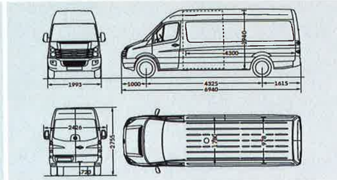
Crafter 50 Kastenwagen langer Radstand mit Hochdach
