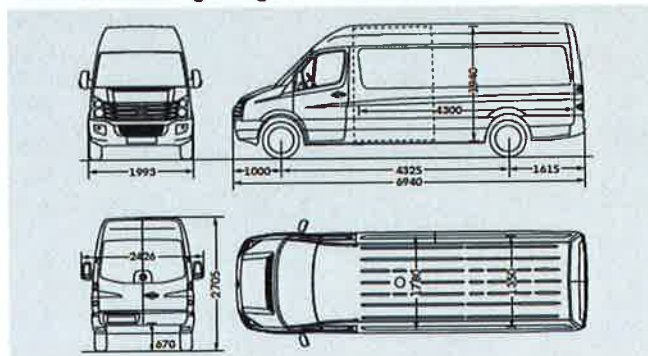
Crafter 35 Kastenwagen langer Radstand mit Hochdach
