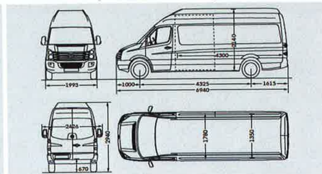
Crafter 35 Kastenwagen langer Radstand mit Superhochdach
