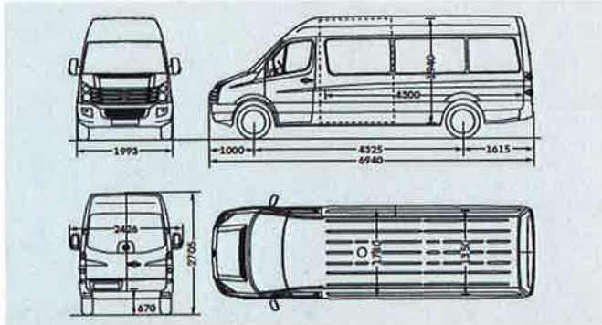
Crafter 35 Kombi langer Radstand mit Hochdach
