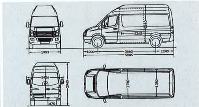
Crafter 35 Kastenwagen mittlerer Radstand mit Superhochdach
