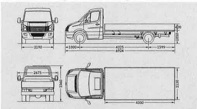
Crafter 50 Pritschenwagen mit Einzelkabine langer Radstand
