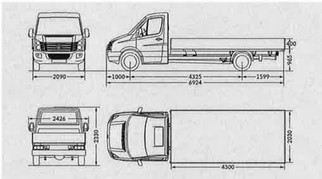
Crafter 35 Pritschenwagen mit Einzelkabine langer Radstand
