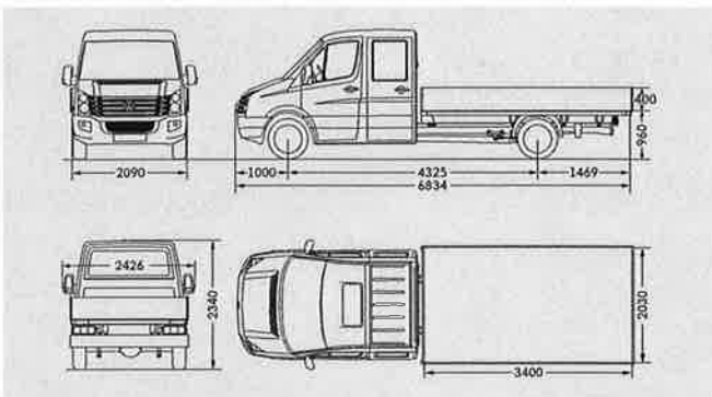
Crafter 35 Pritschenwagen mit Doppelkabine langer Radstand
