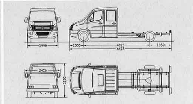
Crafter 35 Fahrgestell mit Doppelkabine langer Radstand
