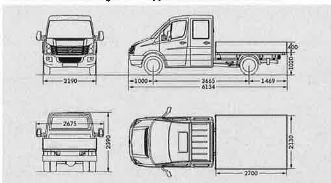
Crafter 50 Pritschenwagen mit Doppelkabine mittlerer Radstand
