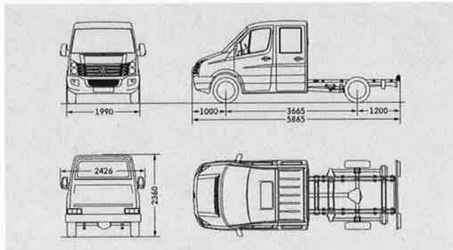
Crafter 35 Fahrgestell mit Doppelkabine mittlerer Radstand
