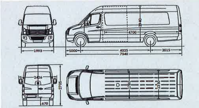
Crafter 35 Kastenwagen langer Radstand mit Überhang mit Hochdach
