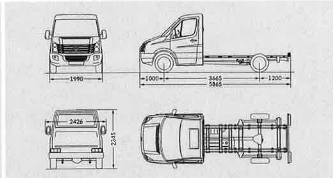
Crafter 35 Fahrgestell mit Einzelkabine mittlerer Radstand
