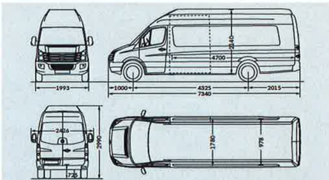
Crafter 50 Kastenwagen langer Radstand mit Überhang mit Superhochdach
