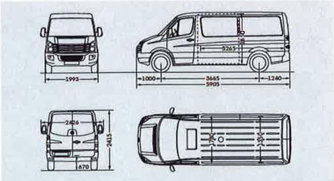
Crafter 30/35 Kombi mittlerer Radstand mit Normaldach
