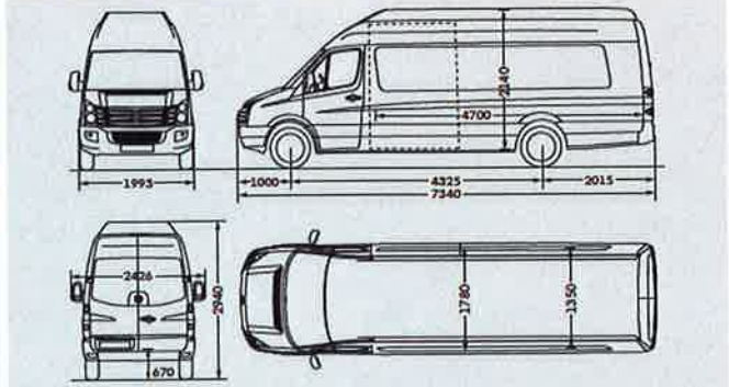
Crafter 35 Kastenwagen langer Radstand mit Überhang mit Superhochdach
