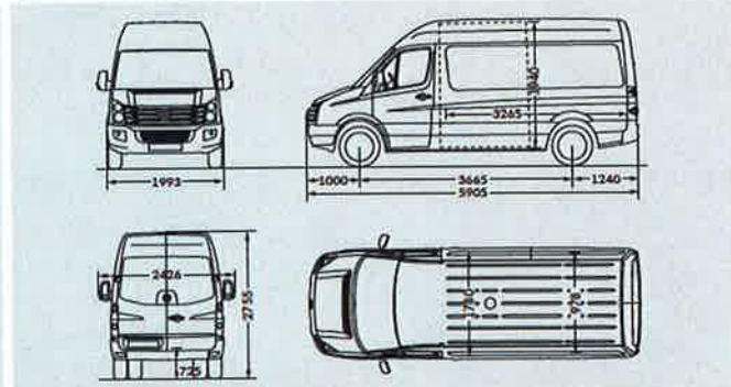
Crafter 50 Kastenwagen mittlerer Radstand mit Hochdach
