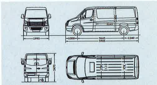
Crafter 50 Kastenwagen mittlerer Radstand mit Normaldach
