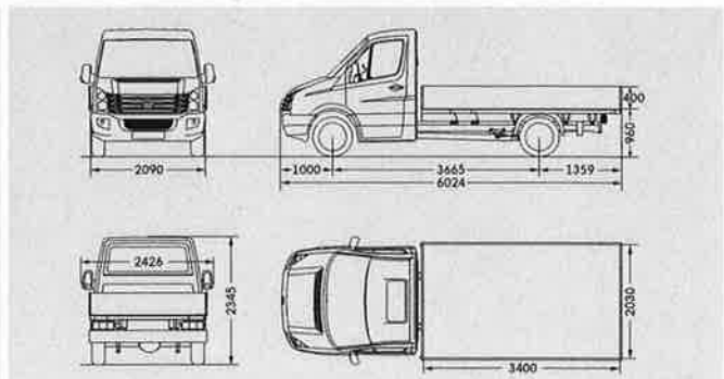
Crafter 35 Pritschenwagen mit Einzelkabine mittlerer Radstand
