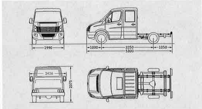
Crafter 30 Fahrgestell mit Doppelkabine kurzer Radstand
