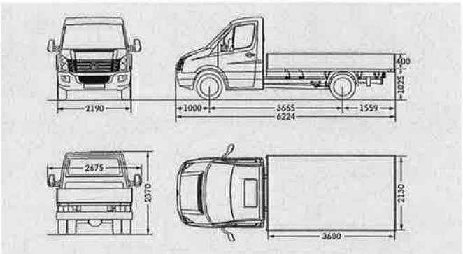
Crafter 50 Pritschenwagen mit Einzelkabine mittlerer Radstand
