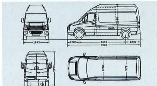
Crafter 50 Kastenwagen mittlerer Radstand mit Superhochdach
