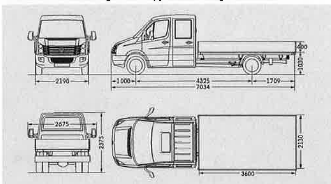
Crafter 50 Pritschenwagen mit Doppelkabine langer Radstand
