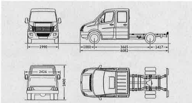
Crafter 50 Fahrgestell mit Doppelkabine mittlerer Radstand
