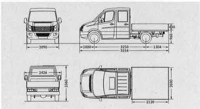
Crafter 35 Pritschenwagen mit Doppelkabine kurzer Radstand
