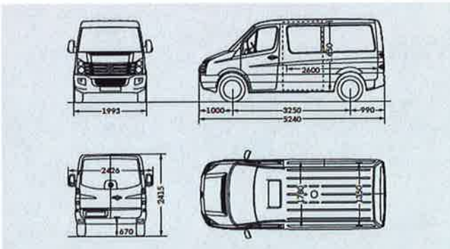
Crafter 30/35 Kombi kurzer Radstand mit Normaldach
