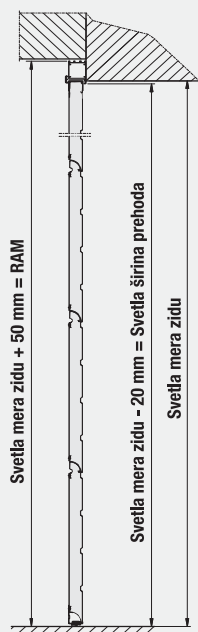
Vgradnja za zidarsko odprtino, odpiranje le navznoter
