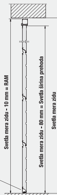
Pozor: Zunanja dimenzija okvirja = Mera za naročilo
