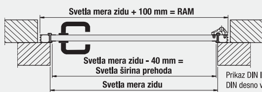
Vgradnja za zidarsko odprtino, odpiranje le navznoter
