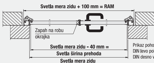
Vgradnja za zidarsko odprtino, odpiranje le navznoter
