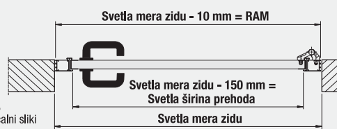
Vgradnja v zidarsko odprtino, odpiranje navznoter ali navzven
