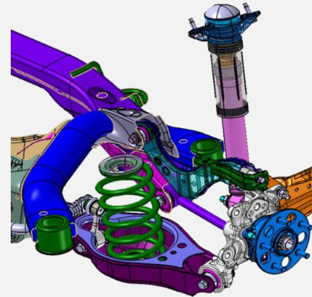
ZADNJE VZMETENJE
