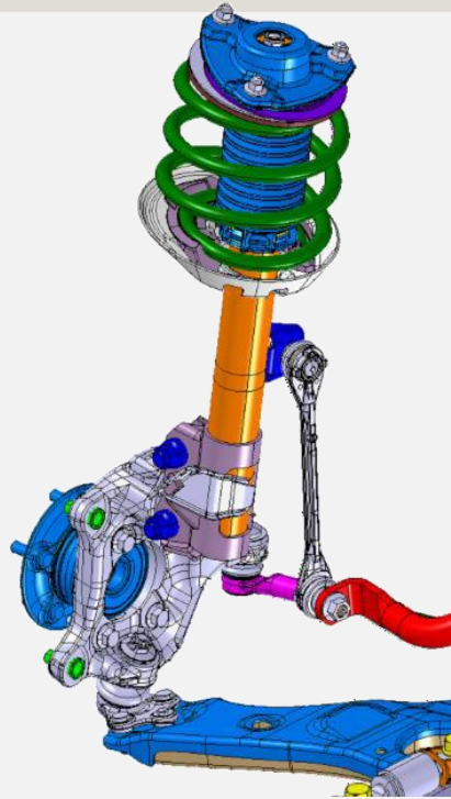
SPREDNJE VZMETENJE
